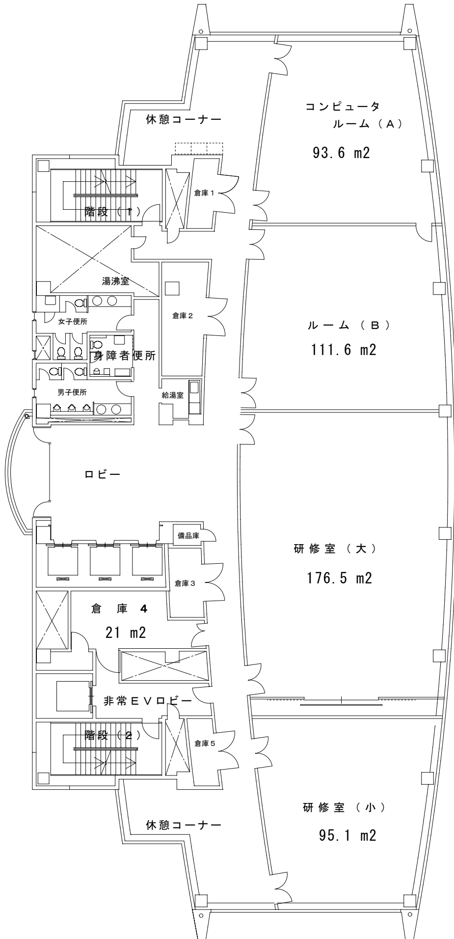
6 階 平面図
